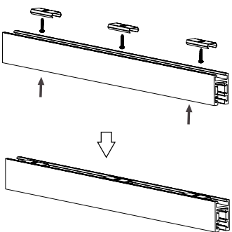
A타입 시공 방법
